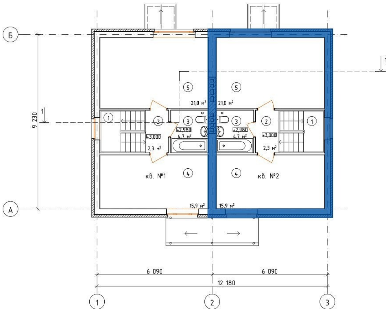
План 2-го этажа на отметке +3.000, М 1:100
